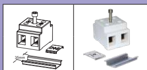
35-mm-Trag-schienenmon-tageclip
